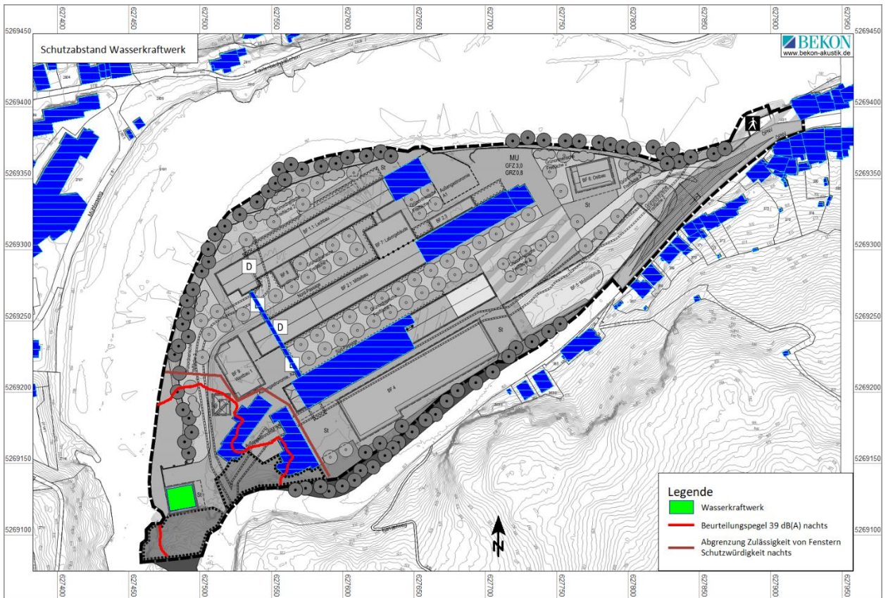
Abbildung 21: Schutzabstand Wasserkraftwerk
